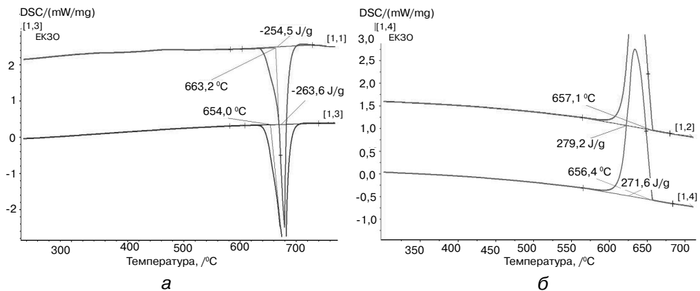
Рис. 1. ДСК-криві алюмінієвого зразка № 1 при нагріванні (а) та охолодженні (б)
