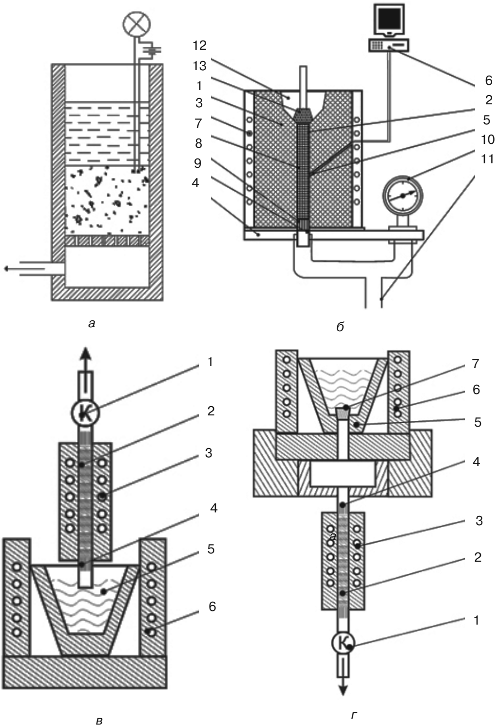
Рис. 1. Схеми установок для просочивання твердих дисперсних частинок металічним розплавом: а – установка для дослідження тиску початку просочивання металевого розплаву через дисперсні частинки; б – установка для дослідження процесів заповнення форми при одержанні композиційних матеріалів методом примусового просочивання, номери окремих вузлів розшифровані у тексті; в, г – установки для одержання литих заготовок методом просочивання з нижньою та верхньою ливниковими системами, відповідно: 1 – вакуумний кран; 2 – дисперсні частинки; 3 – піч опору; 4 – пориста керамічна вставка; 5 – розплав; 6 – плавильна піч; 7 – графітова заглушка (стопор)
