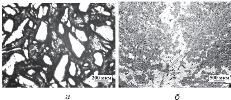
Рис. 6. Мікроструктура композиту на основі алюмінієвого сплаву АК12 з 60 об. % дисперсних частинок ВК8: а – одержаний методом вакуумного просочування; б – одержаний розчиненням частинок твердого сплаву в розплаві при температурі 1200 °С і часі витримки 30 хв
