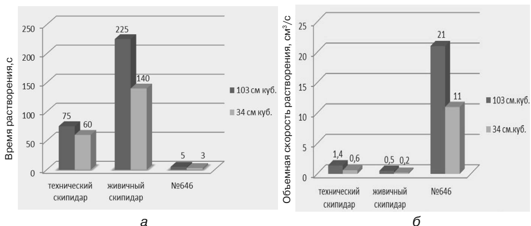
Рис. 1. Влияние видов растворителя на время растворения и объемную скорость блочного ППС; \rho = 25 \text{ кг/м}^3 (серое); \rho = 35 \text{ кг/м}^3 (черное)
