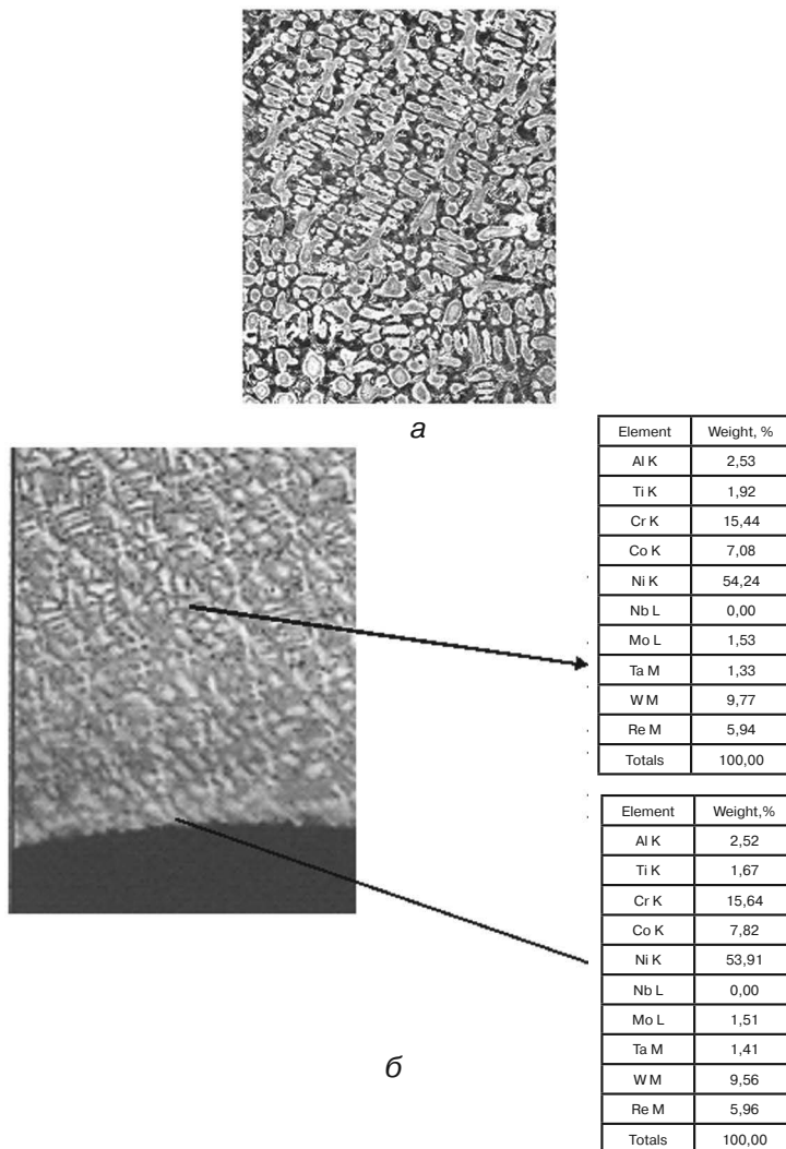
Рис. 4. Металлографические исследования полученных образцов разработанного сплава: а – макроструктура сплава (равноосное состояние), \times 50 ; б – поперечное сечение в состоянии НК ( \gamma - твердый раствор), \times 200
