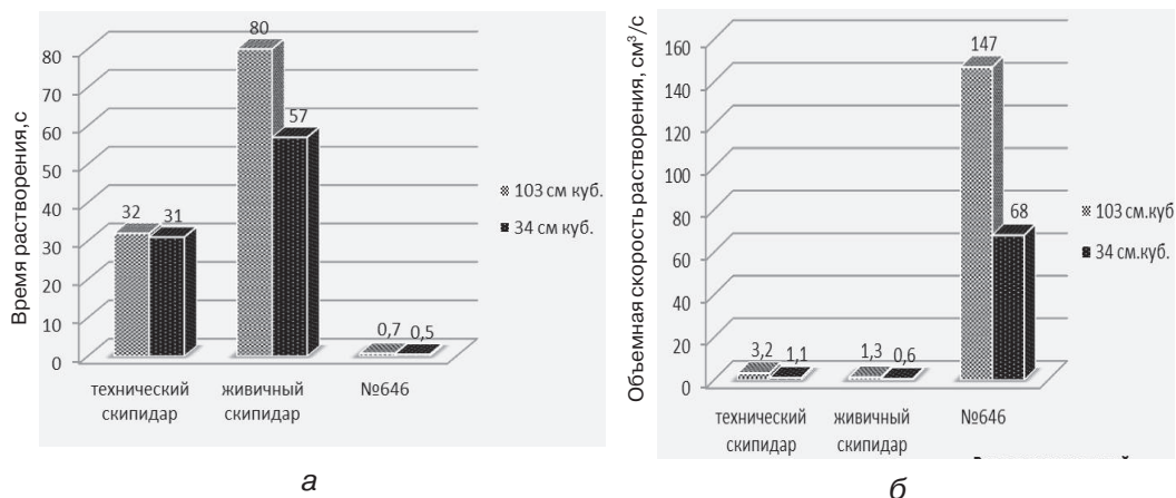
Рис. 2. Влияние видов растворителя на время растворения и объемную скорость экструдированного ППС; \rho = 25 \text{ кг/м}^3 (серое); \rho = 35 \text{ кг/м}^3 (черное)
