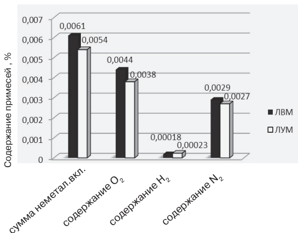
Рис. 3. Сравнительная характеристика чистоты приповерхностной зоны (по содержанию газов) в отливках, полученных методом ЛВМ и ЛУМ для жаропрочного сплава
