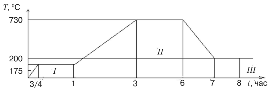
Рис. 2. Режим прокаливания формы: I – нагрев и выплавка модельного состава; II – нагрев и прокаливание формы; III – подготовка формы под заливку
