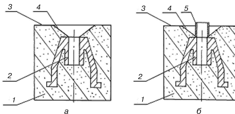
Рис. 2. Литейная форма: в разрезе по оси цилиндра отливки (а); то же с патрубком, установленном на отливке (б): 1 – песок; 2 – цилиндр (гильза) отливки блока цилиндров; 3 – контрлад; 4 – естественный откос песка; 5 – патрубок
