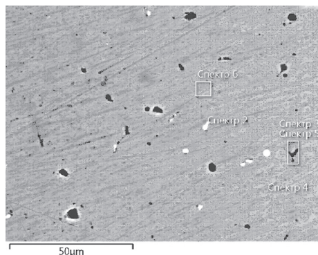
Рис. 5. Результаты РСМА фрагмента образца
