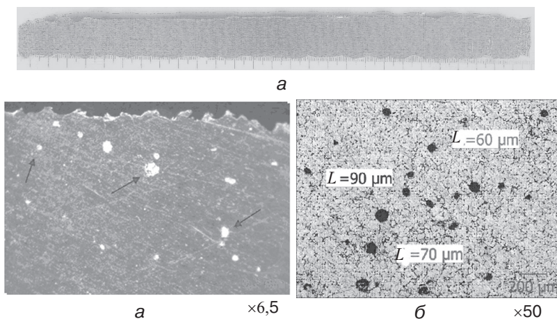
Рис. 3. Макроструктура наплавленного образца
