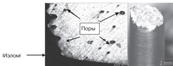
Рис. 2. Микрошлиф с выходом на излом у образца № 1
