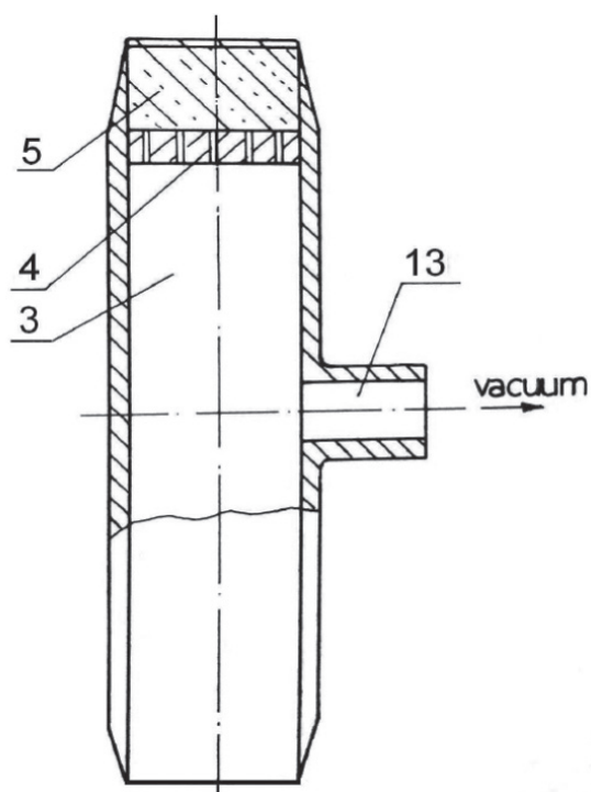
Рис. 3. Роторно-конвейерное устройство для непрерывного получения полосы из расплава
