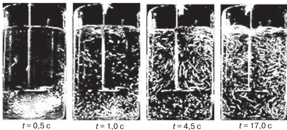
Рис. 5. Видеограмма процесса перемешивания турбинной мешалкой в режиме реверса 1/1, H = 42 мм, n = 400 об/мин
