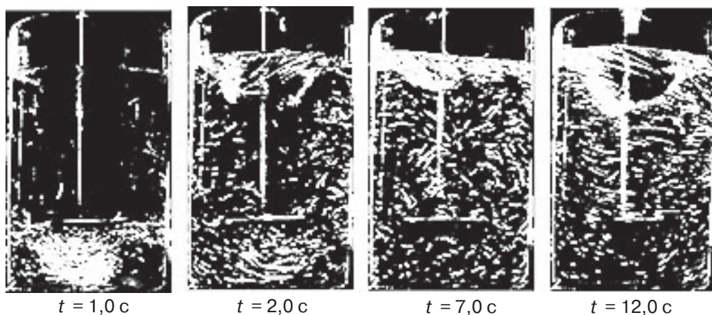
Рис. 6. Видеограмма процесса перемешивания турбинной мешалкой в реверса 3/3, H = 42 мм, n = 400 об/мин
