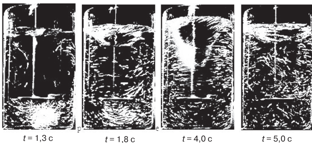
Рис. 7. Видеограмма процесса перемешивания турбинной мешалкой в режиме реверса 5/5, H = 42 мм, n = 400 об/мин
