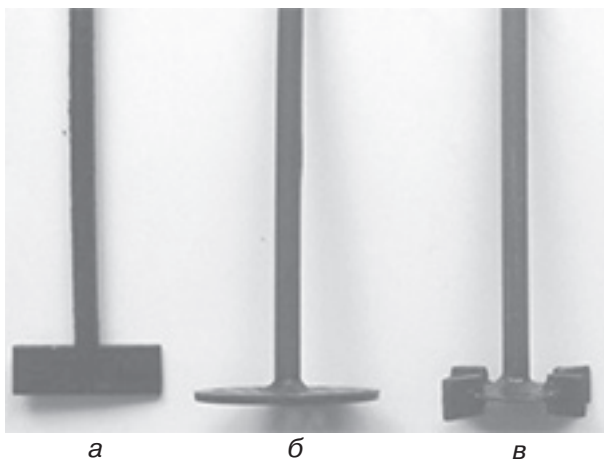
Рис. 1. Типы мешалок, используемых для натурных исследований: а – лопастная; б – дисковая; в – турбинная
