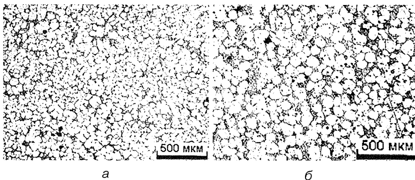
Рис. 3. Исследование процесса тиксолитья сплава АК7ч с использованием заготовок с исходной глобулярной структурой первичной фазы: а – исходная структура заготовки; б – структура, которая образуется в фасонной отливке после тиксолитья
