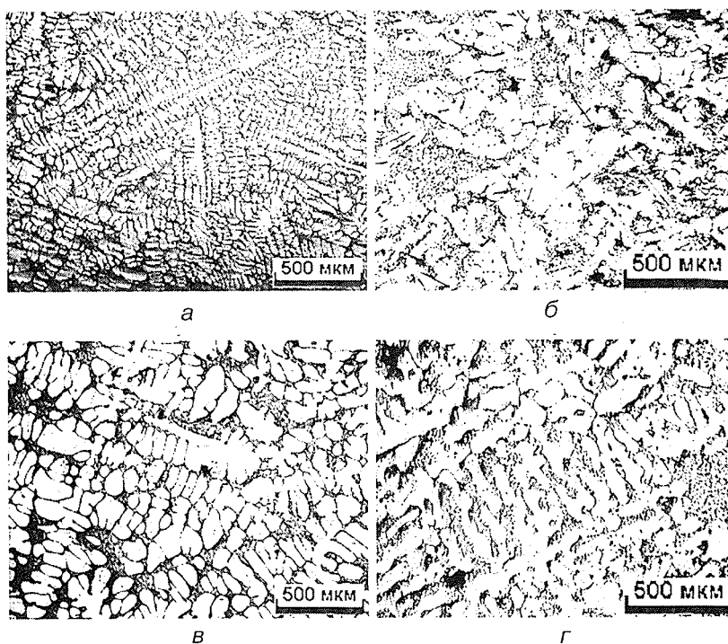
Рис. 1. Исследование процесса тиксолития сплава АК74 с использованием заготовок с исходной дендритной структурой первичной фазы: а, в – исходные структуры в заготовках; б, г – структуры, которые образовались в отливках
