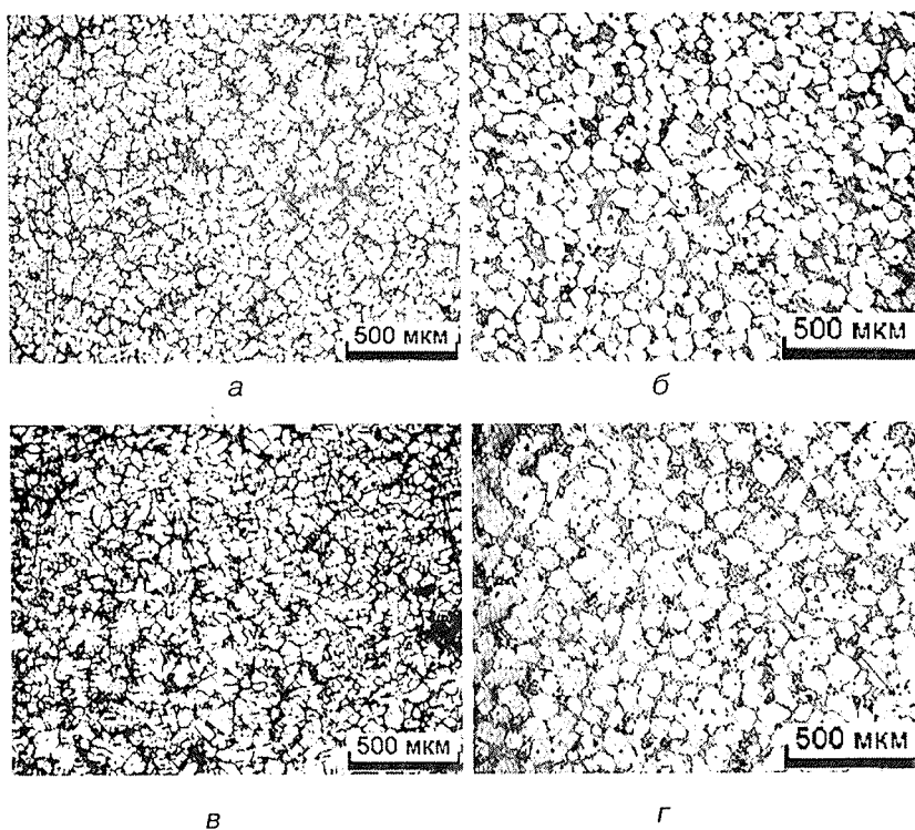
Рис. 2. Исследование процесса тиксолития сплава АК74 с использованием заготовок с исходной розеткоподобной структурой первичной фазы: а, в – исходная структура заготовок; б, г – структуры, которые образовались в фасонных отливках после тиксолития
