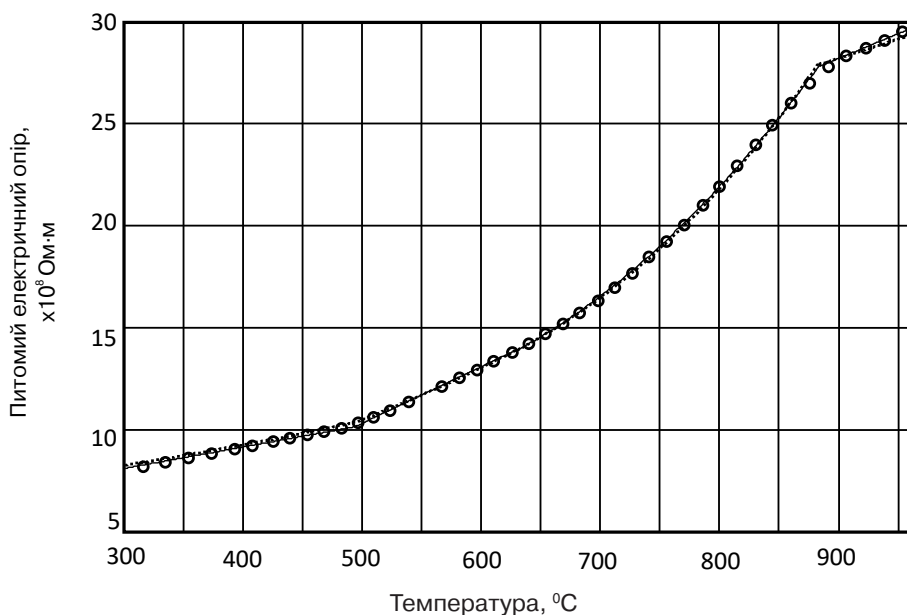
Рис. 1. Температурна залежність питомого електричного опору бронзи К1НЗ: – за о – експериментальними даними; . . . . . – розрахована за виразом (2)
